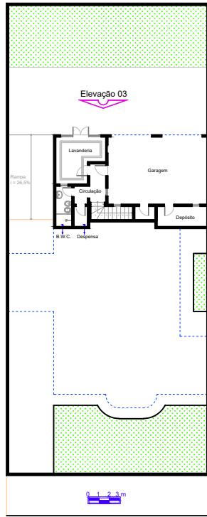
Subsolo A = 77,50 m 2
