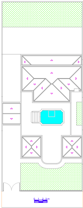
Implantação e Cobertura
