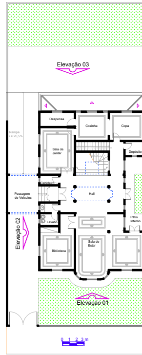
Térreo A = 197,74 m 2
