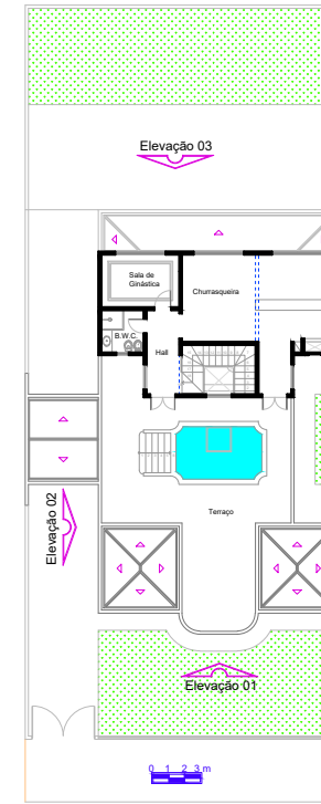
Cobertura A = 69,50 m 2
